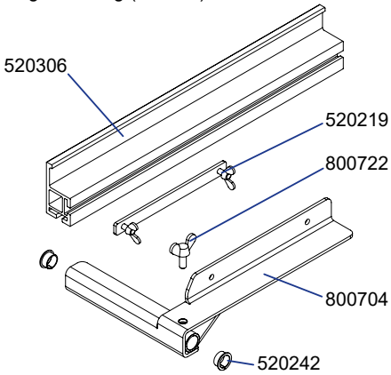
Längsanschlag (800703)
